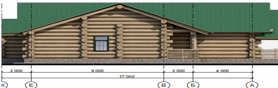
ФАСАД Ж-А
